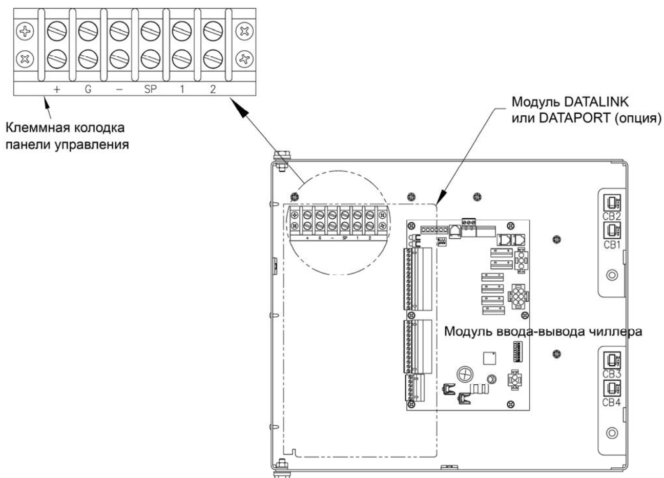
РАСПОЛОЖЕНИЕ КОМПОНЕНТОВ ПАНЕЛИ УПРАВЛЕНИЯ
