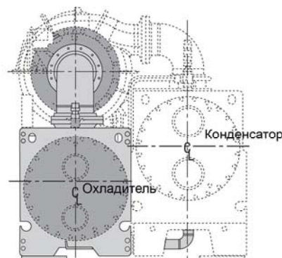
ВИД С ТОРЦА
