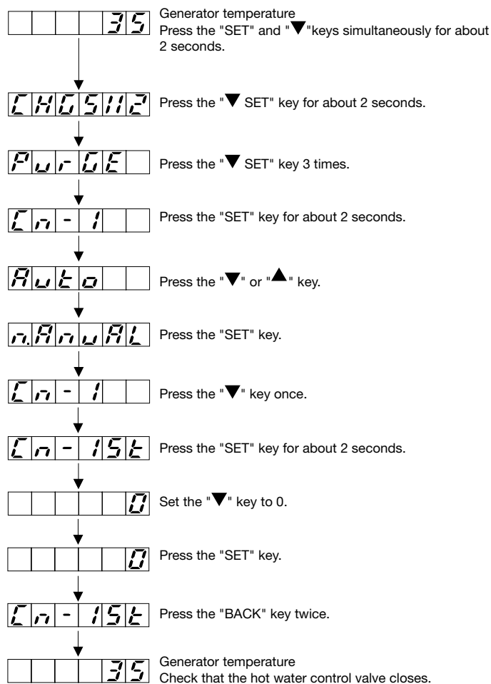
Fig. 8 - Display example
